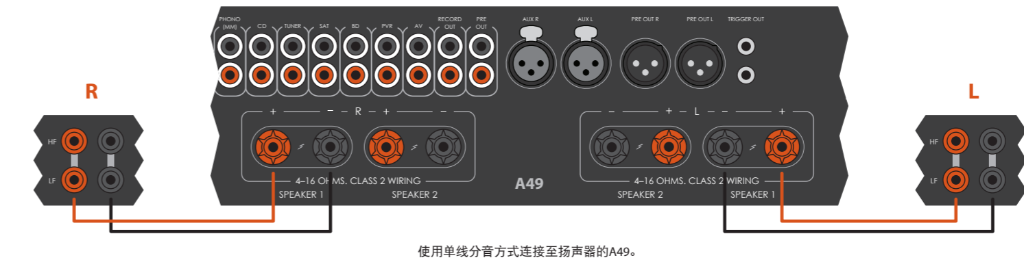
使用单线分音方式连接至扬声器的A49。
