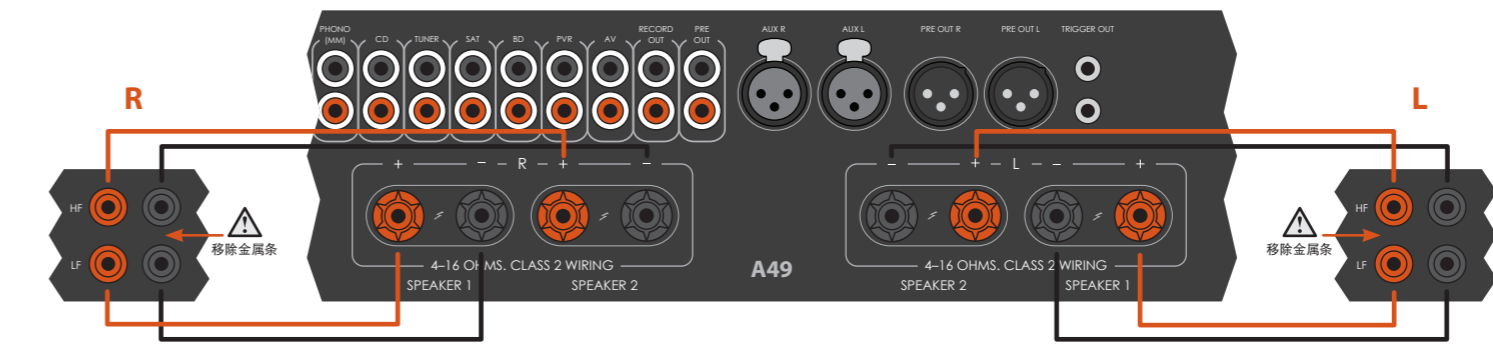
使用双线分音方式连接至两组扬声器的A49。
